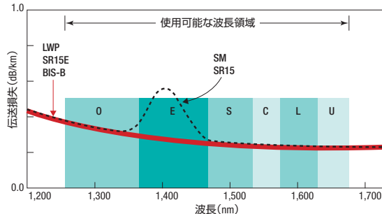
広帯域伝送シングルモードファイバ
